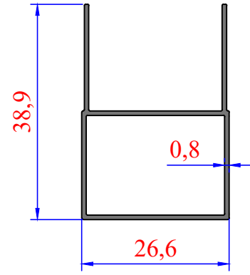
3279 0,277 kg/m 28'lik Plice Kasa
