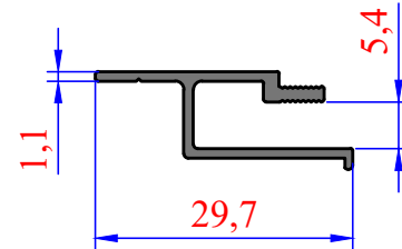
3243 0,182 kg/m Gergi Tavan
