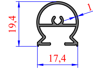
3494 0,224 kg/m Bella Seri
