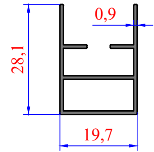
3967 0,253 kg/m 19'luk Plice Kasa
