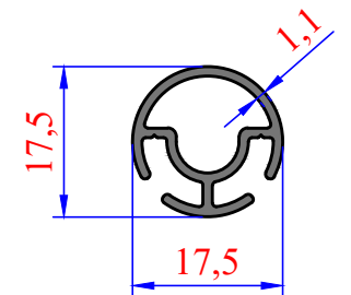
3661 0,209 kg/m
