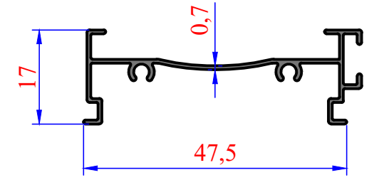
3003 0,233 kg/m Zebra Geniş Kasa
