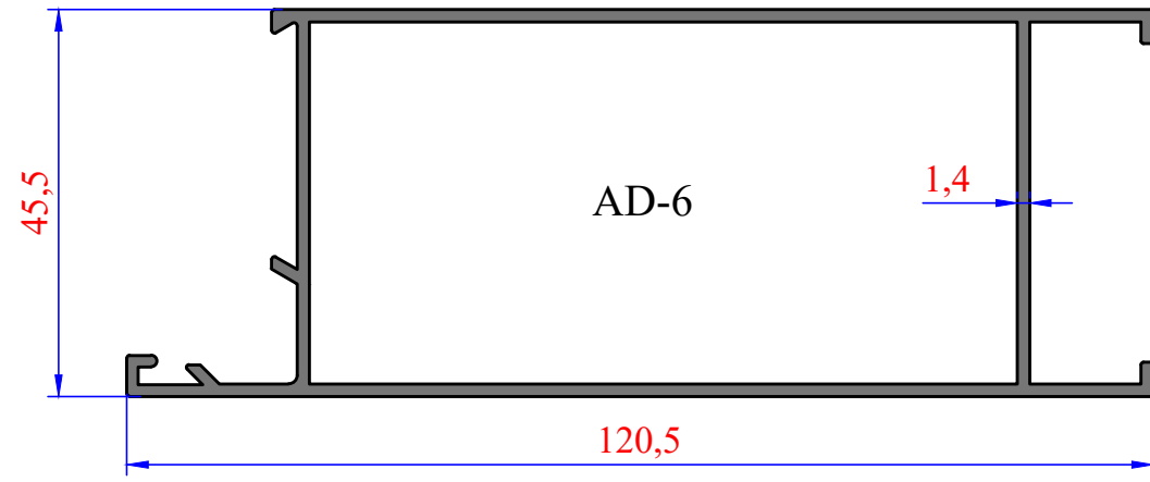
3397 1,283 kg/m ALDOKS ETEK
