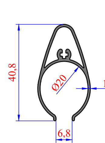
3041 0,345 kg/m Armut Lama
