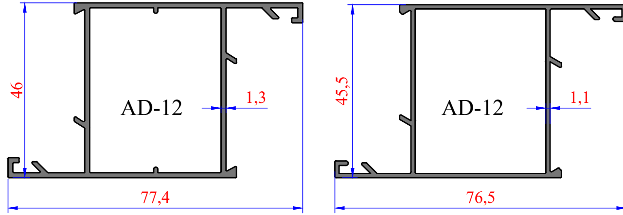
3455 0,841 kg/m AD Z KANAT
