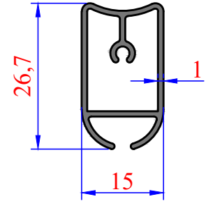
3522 0,263 kg/m Kanallı Lama
