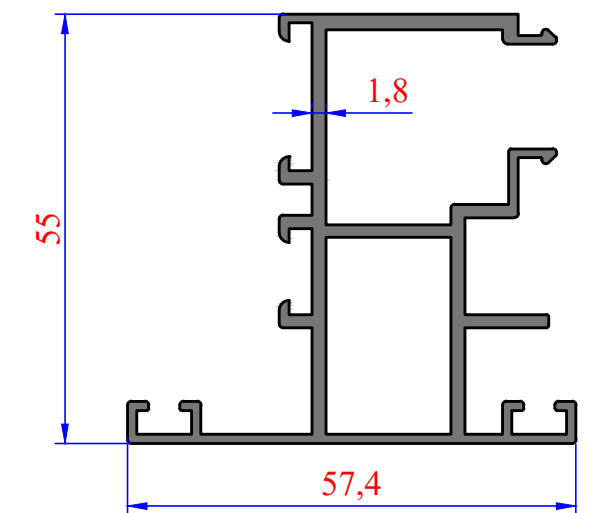
3444 1,107 kg/m SİSTEM ÇİFT KAPI ADAPTÖR
