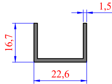
3549 0,217 kg/m
