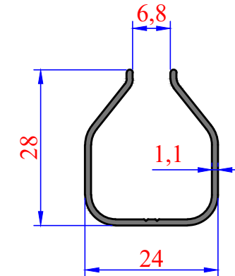
3660 0,233 kg/m
