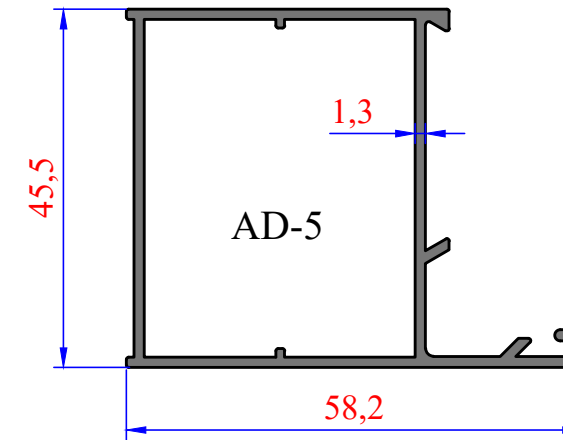
3398 0,718 kg/m AD YARIM SERİ KASA
