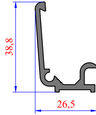
3683 0,449 kg/m Sürme Kilit 2
