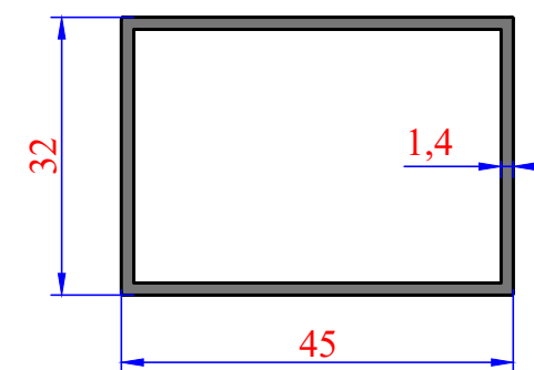
4049 0,563 kg/m
