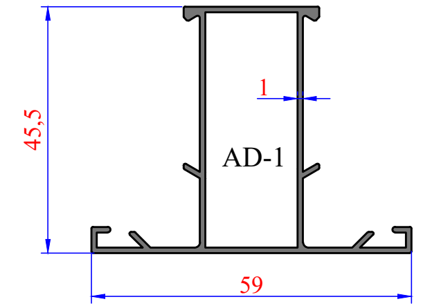
3225 0,556 kg/m AD DAR ORTA KAYIT
