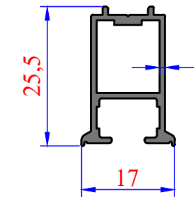
3497 0,249 kg/m Bella Seri
