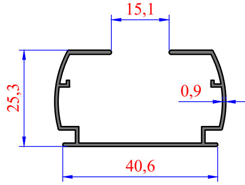
3021 0,325 kg/m
