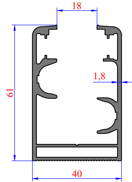
3202 1,255 kg/m Firtına Kasa
