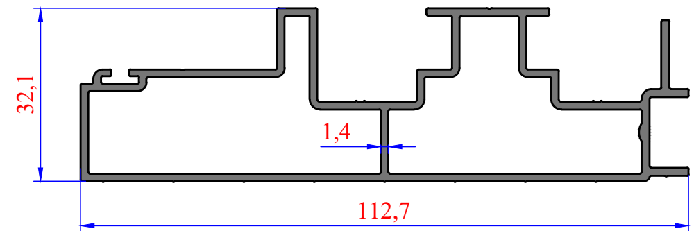
3861 1,372 kg/m
