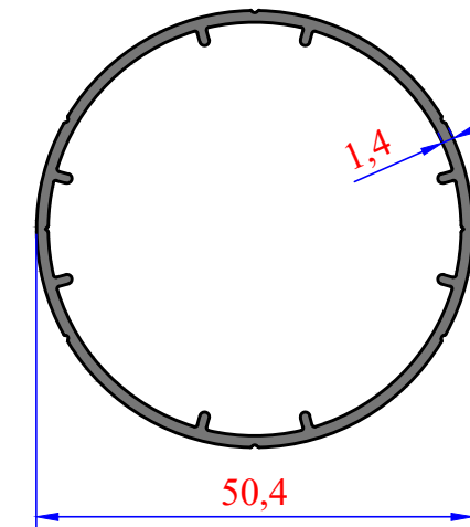
3108 0,605 kg/m
