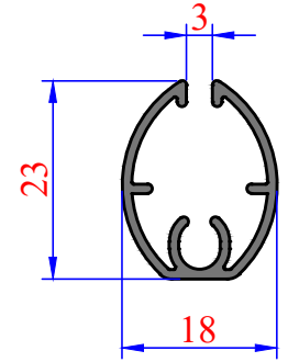
3525 0,240 kg/m
