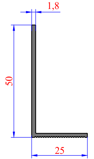
3214 0,347 kg/m
