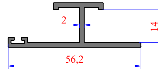
3212 0,528 kg/m
