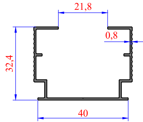
3032 0,357 kg/m
