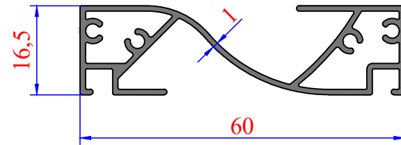
3436 0,552 kg/m
