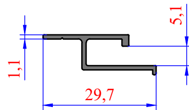
3242 0,158 kg/m Gergi Tavan
