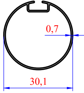
3011 0,196 kg/m 30'luk Stor Boru
