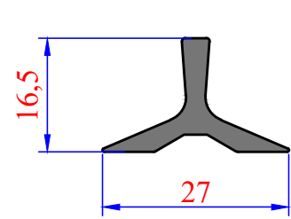
3708 0,290 kg/m Cetvel
