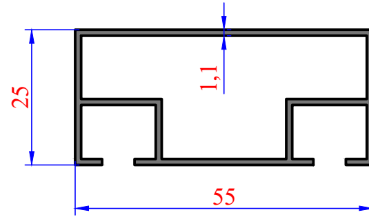
3559 0,577 kg/m
