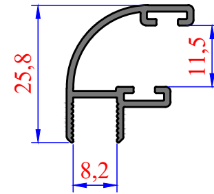
3693 0,266 kg/m 90° Fitol
