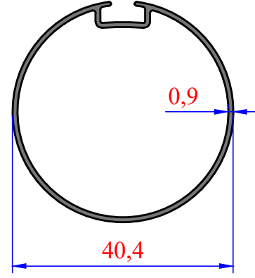
3037 0,325 kg/m 38'lik Jumbo Tırnaksız
