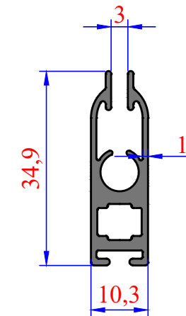
3524 0,387 kg/m
