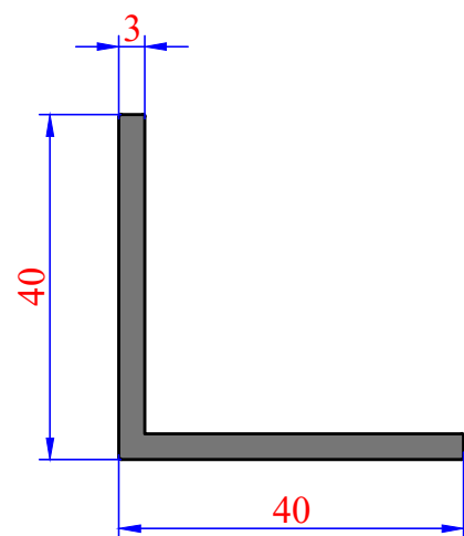
3726 0,626 kg/m
