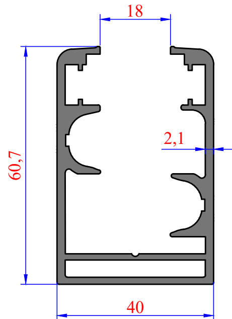
3256 1,464 kg/m Firtına Kasa
