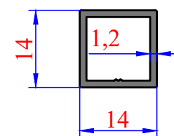
3612 0,166 kg/m
