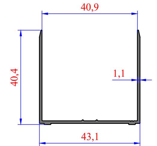
3964 0,363 kg/m
