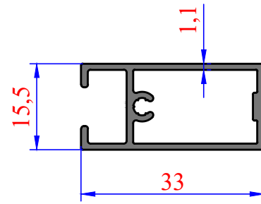
3499 0,340 kg/m Bella Seri
