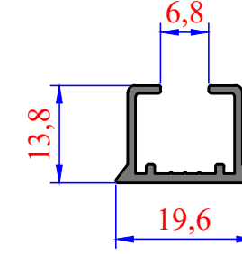
3067 0,174 kg/m
