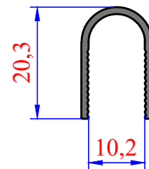
3602 0,154 kg/m 10mm U Fitol
