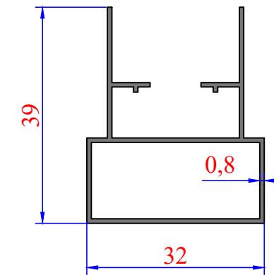
3277 0,333 kg/m 32'lik Plise Kasa
