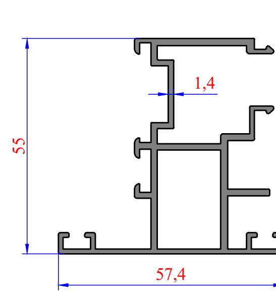
4048 1,075 kg/m SİSTEM ÇİFT KAPI ADAPTÖR
