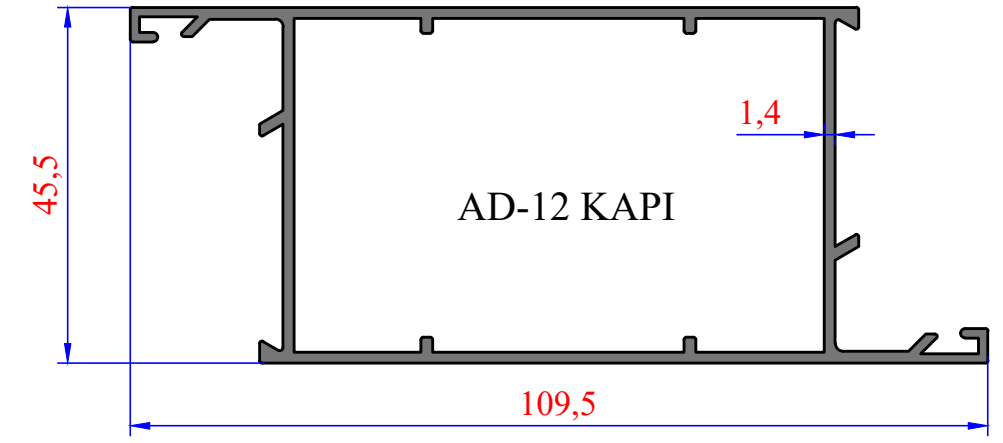
3400 1,153 kg/m AD GENİŞ KAPI
