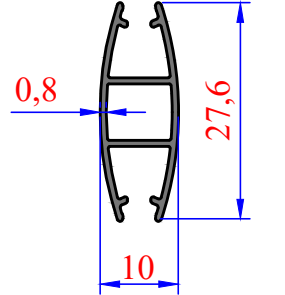
3034 0,168 kg/m Stor Etek Çıtası
