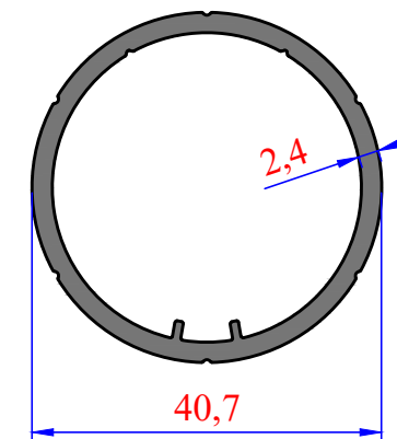
3835 0,776 kg/m
