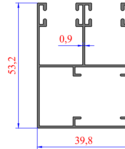
3267 0,680 kg/m
