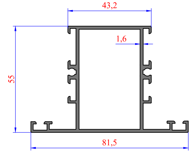
3446 1,221 kg/m SİSTEM 2 ORTA KAYIT
