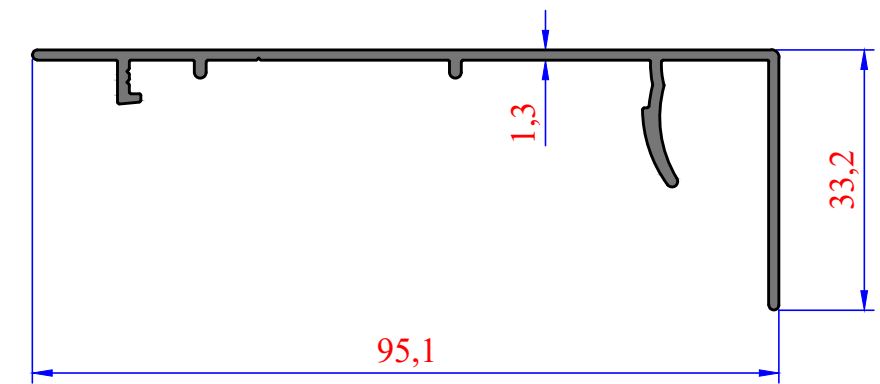
3715 R1 0,563 kg/m
