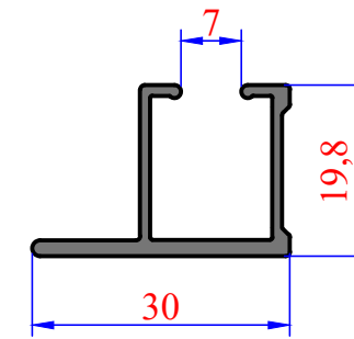
3703 0,297 kg/m
