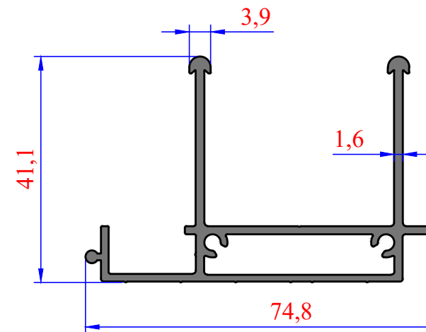
3983 0,904 kg/m
