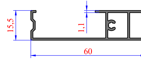
3493 0,439 kg/m Bella Seri
