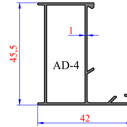
3224 0,464 kg/m AD DAR KASA
