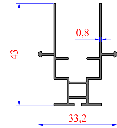
3278 0,341 kg/m 32'lik Plise Kanat
