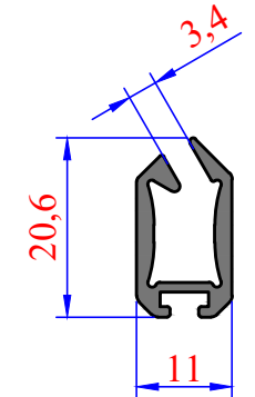
3044 0,233 kg/m Özel Lama
