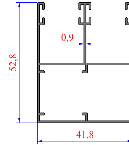
3234 0,639 kg/m
