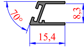
3287 0,118 kg/m 22,5° Fitol
