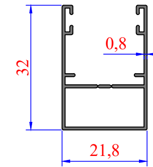
3237 0,249 kg/m
