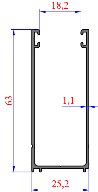
3096 0,477 kg/m
