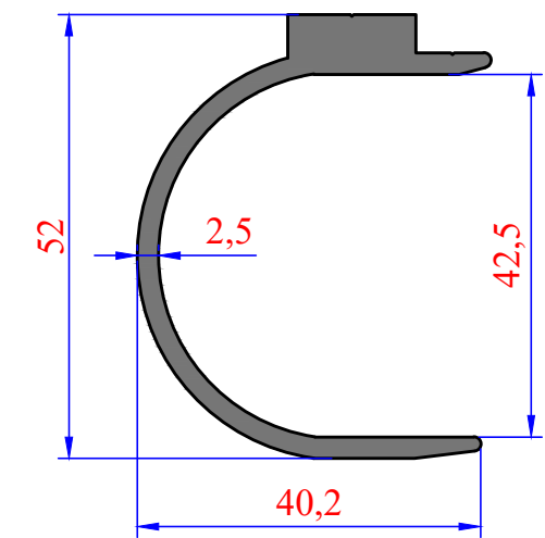
3052 0,880 kg/m 4cm'lik Rustik Ayağı
