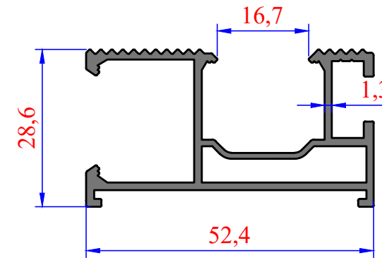
3924 0,711 kg/m
