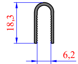
3632 0,131 kg/m 6mm U Fitol
