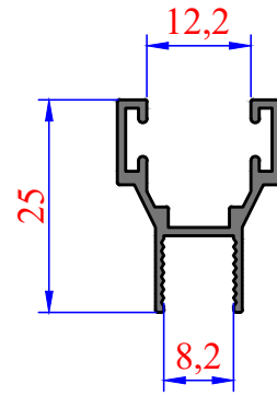
3240 0,220 kg/m Büyük H
