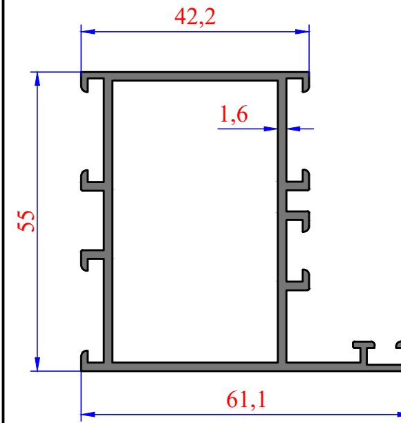
3443 1,068 kg/m SİSTEM 5 KASA
