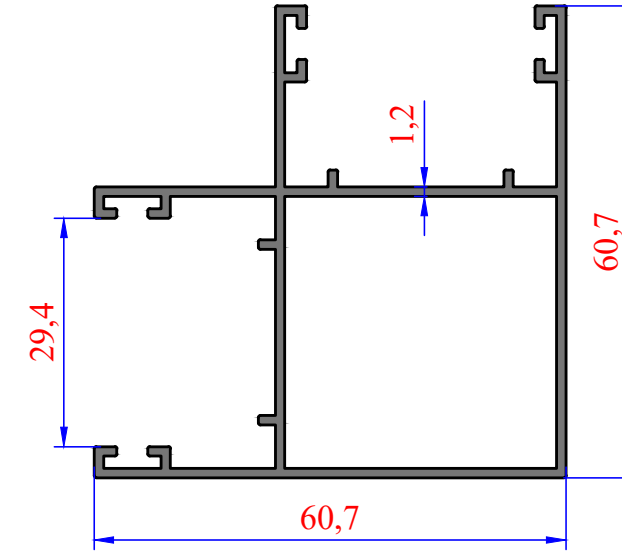
3457 0,918 kg/m Sürme 90° Köşe
