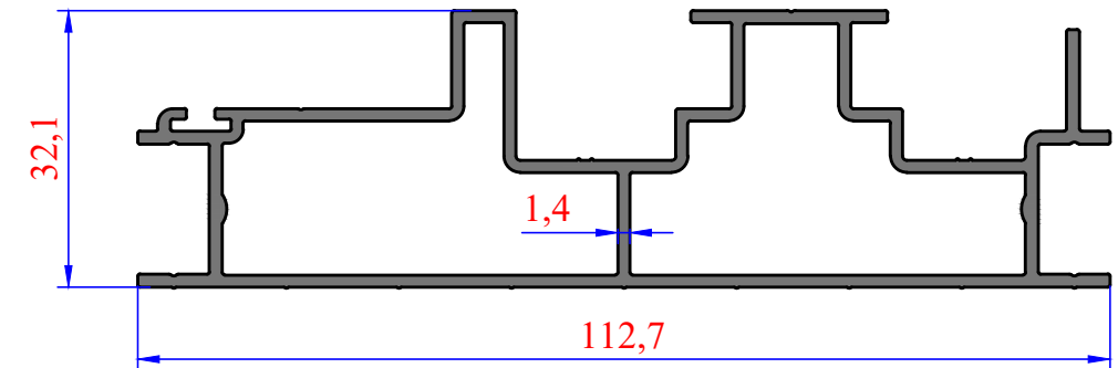
3863 1,384 kg/m
