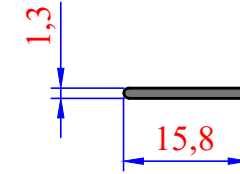
3555 0,055 kg/m Lazer Perde Mili
