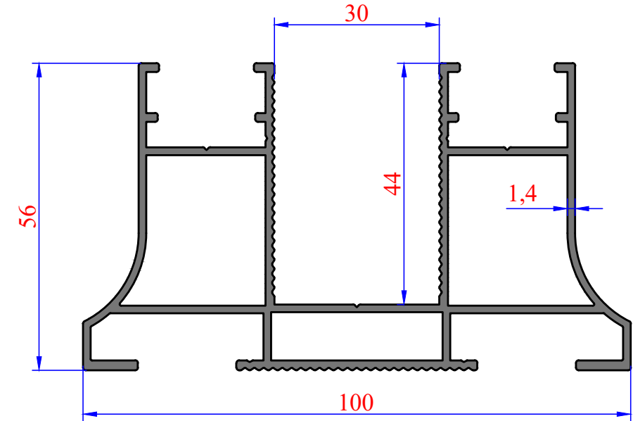
3644 1,697 kg/m
