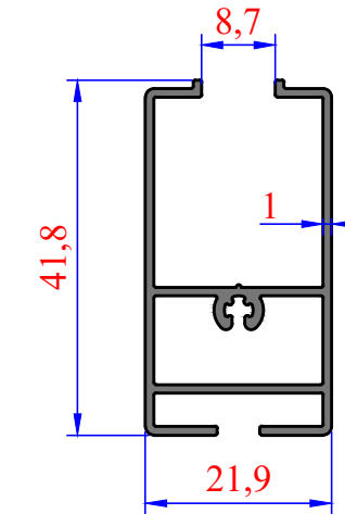
3043 0,444 kg/m Özel Lama
