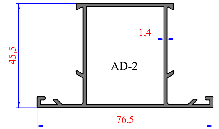
3399 0,878 kg/m AD YARIM SERİ ORTA KAYIT
