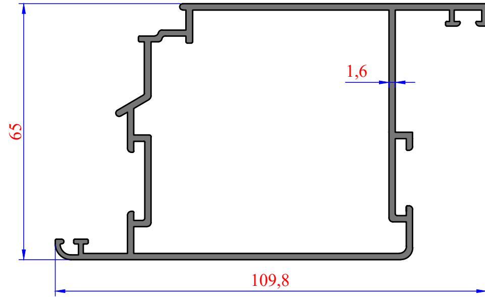
3441 1,534 kg/m SİSTEM GENİŞ KAPI
