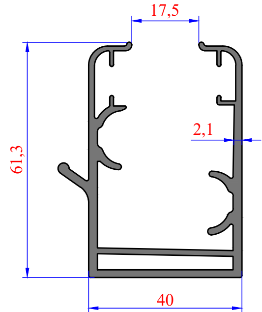
3290 1,336 kg/m Gold Kasa Oluklu
