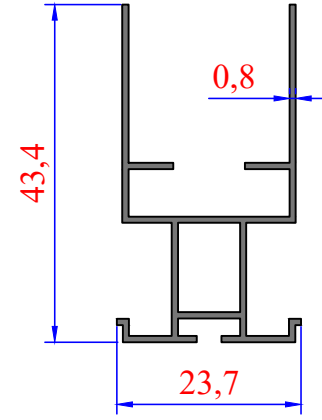
3280 0,326 kg/m 28'lik Plice Kanat
