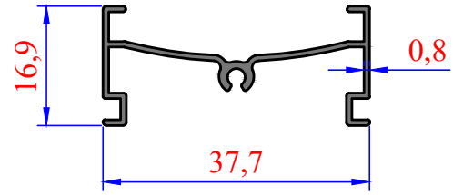
3001 0,207 kg/m Dar Stor Kasa
