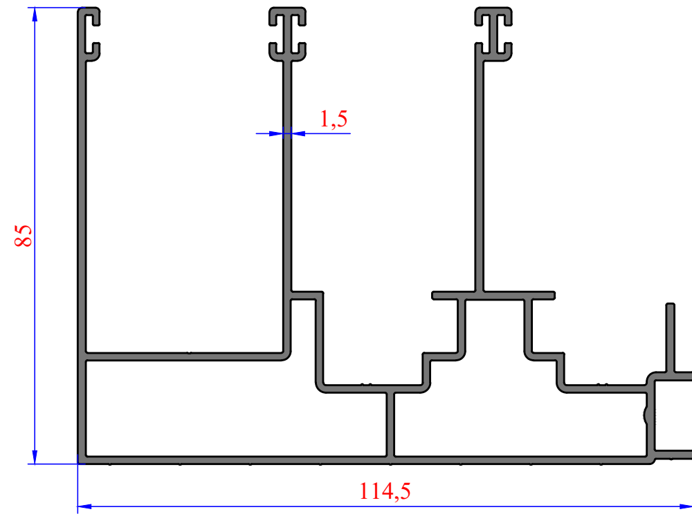
3860 2,213 kg/m
