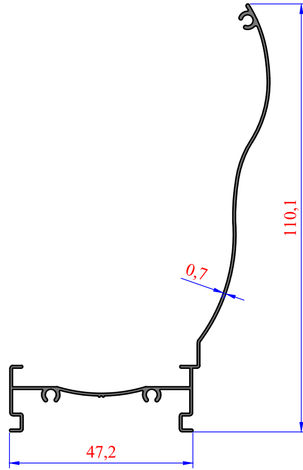
3113 0,426 kg/m Çiftli Kapalı Kasa
