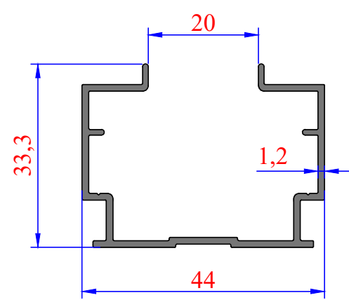
3731 0,449 kg/m
