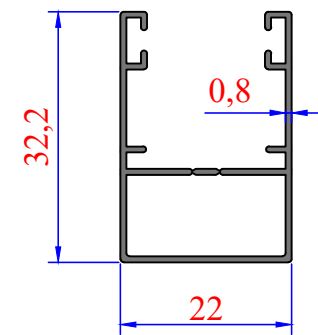
3339 0,257 kg/m
