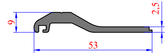
3925 0,504 kg/m
