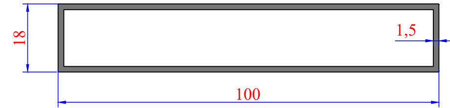
3551 0,936 kg/m
