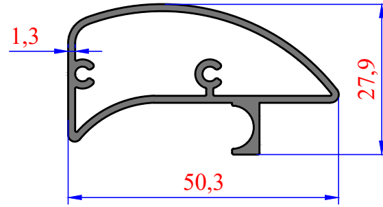
3997 0,579 kg/m Lüks Seri
