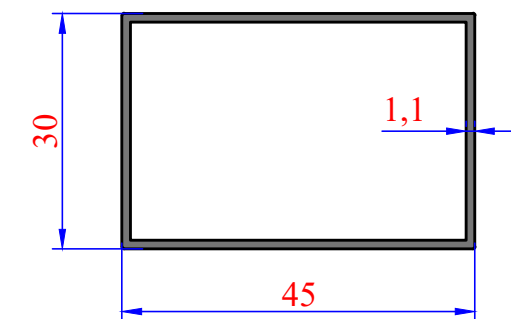
3801 0,434 kg/m
