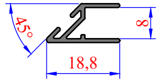
3286 0,128 kg/m 45° Fitol
