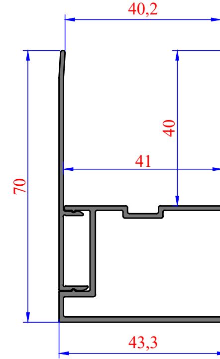
3598 - 3599 0,872 kg/m
