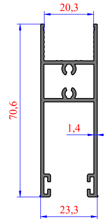
3986 0,804 kg/m
