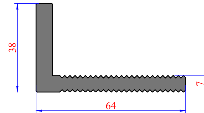
3926 1,668 kg/m
