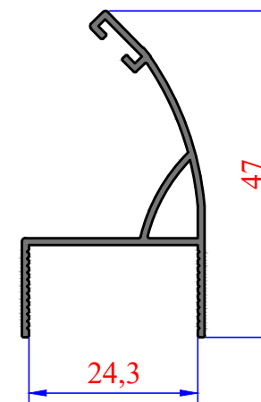
3694 0,297 kg/m 45° ISICAM FİTİL
