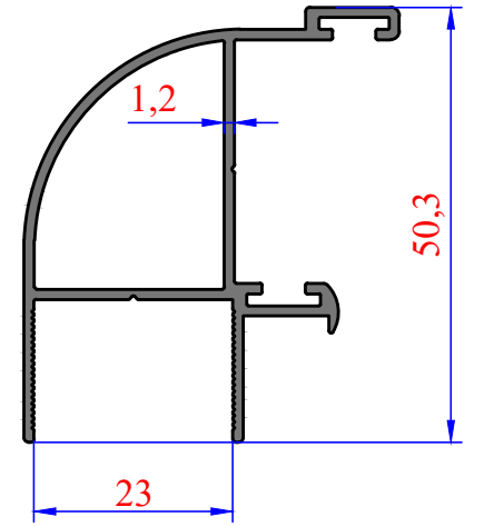
3704 0,565 kg/m Sürme 90° Köşe
