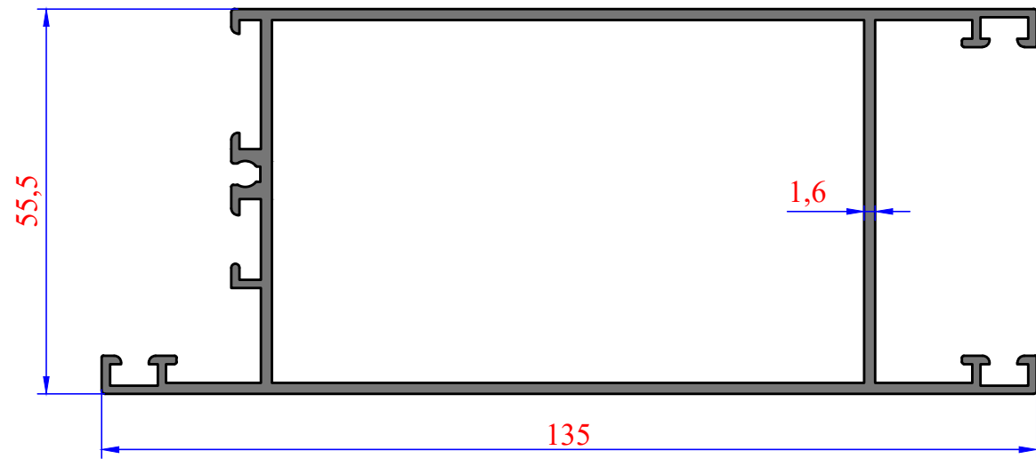
3440 1,725 kg/m SİSTEM 135'lik ETEK
