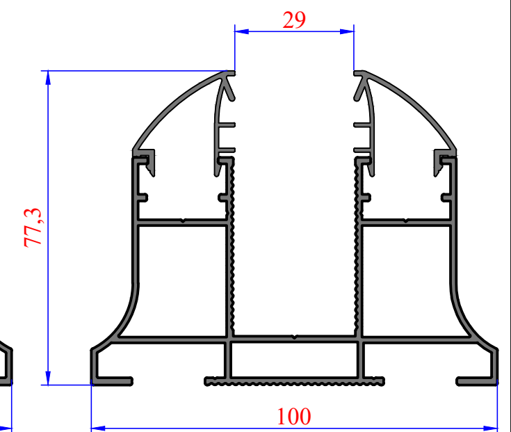
3646 0,334 kg/m
