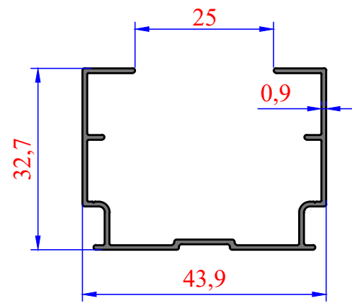
3697 0,312 kg/m
