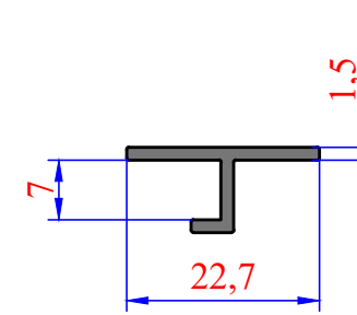
3209 0,141 kg/m
