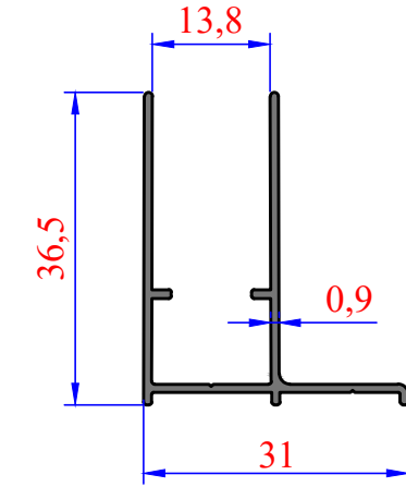
3496 0,278 kg/m Bella Seri
