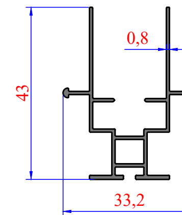
3981 0,345 kg/m 32'lik Plise Kanat
