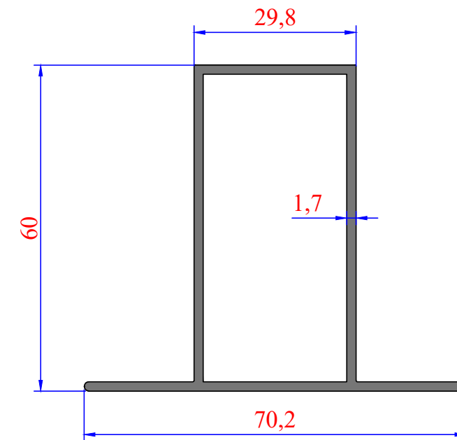
3564 0,982 kg/m
