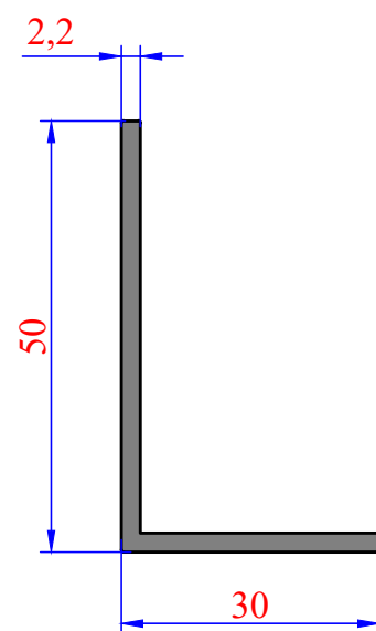
3969 0,464 kg/m
