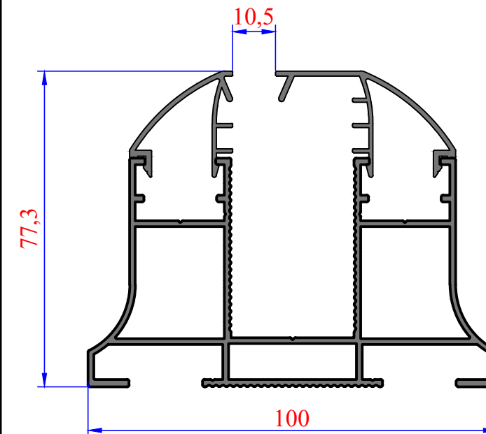
3645 0,256 kg/m
