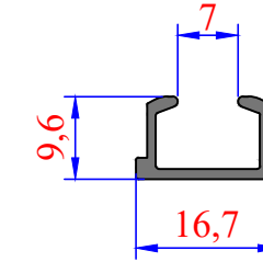
3782 0,125 kg/m
