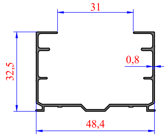
3532 0,325 kg/m
