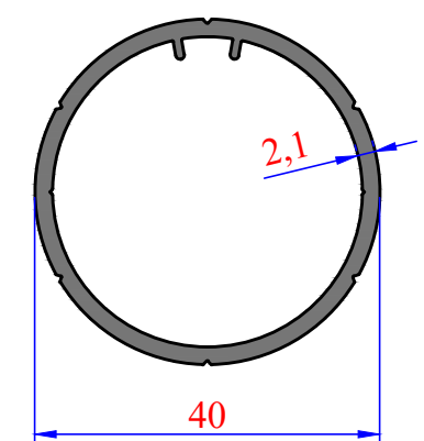
3106 0,670 kg/m
