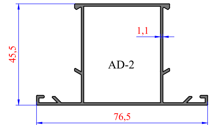
3935 0,710 kg/m AD YARIM SERİ ORTA KAYIT
