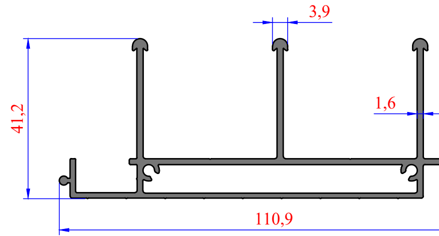
3982 1,321 kg/m
