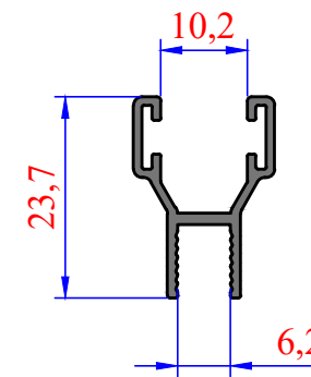
3630 0,202 kg/m 6mm Büyük H
