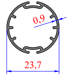
3235 0,238 kg/m
