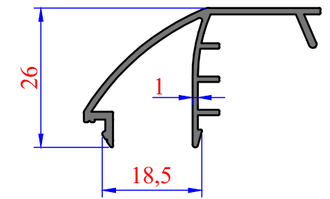
3646 0,334 kg/m
