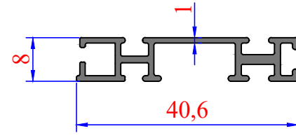
3337 0,276 kg/m
