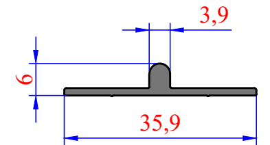
3987 0,180 kg/m
