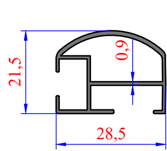
3065 0,289 kg/m
