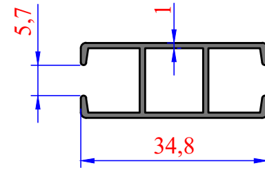
3047 0,290 kg/m Hastane Rayı
