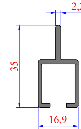
3342 0,333 kg/m
