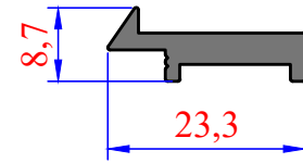
3684 0,229 kg/m Sürme Kilit Karşılığı
