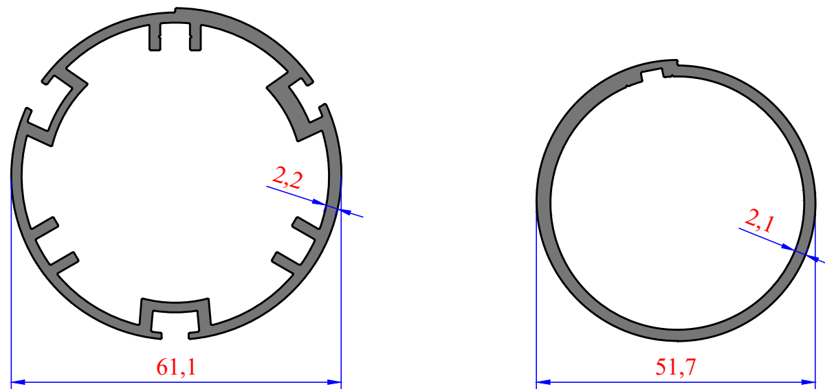
3712 1,419 kg/m
