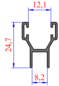
3797 0,213 kg/m Büyük H
