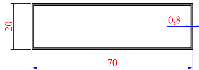
3448 0,382 kg/m
