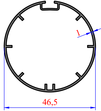
3013 0,470 kg/m 47'lik Motor Boru
