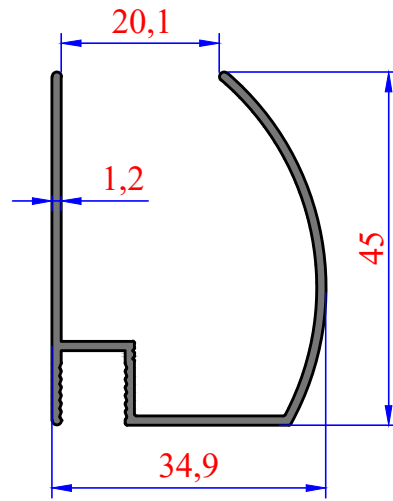
3998 0,423 kg/m Lüks Seri
