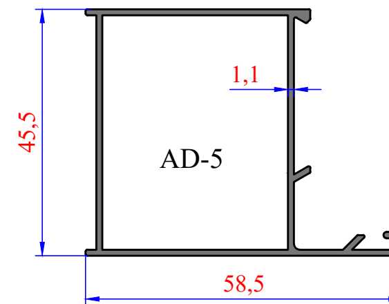
3934 0,604 kg/m AD YARIM SERİ KASA
