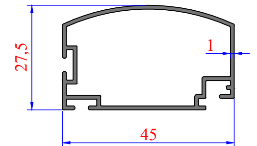
3269 0,436 kg/m
