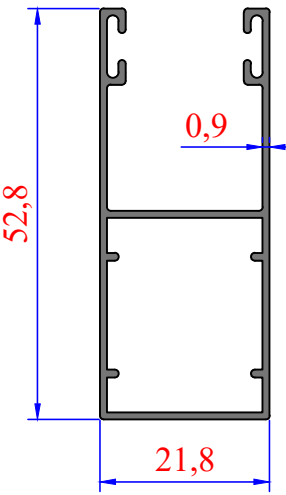
3233 0,417 kg/m
