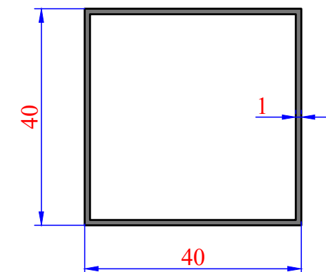
3259 0,422 kg/m
