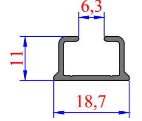
3727 0,147 kg/m
