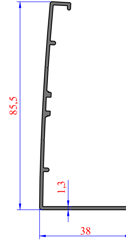
3714 0,506 kg/m
