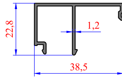
3445 0,304 kg/m SİSTEM TEK CAM ÇITA
