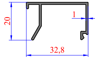
3936 0,250 kg/m AD ÇITA 6mm
