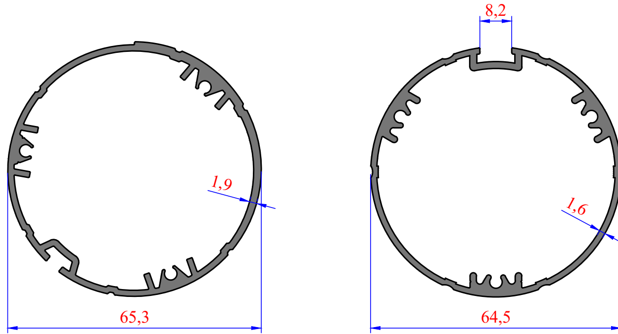
3711 1,245 kg/m
