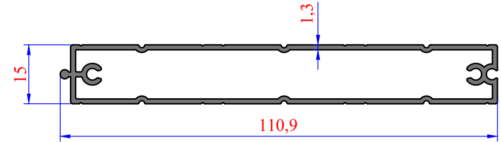
3984 0,920 kg/m
