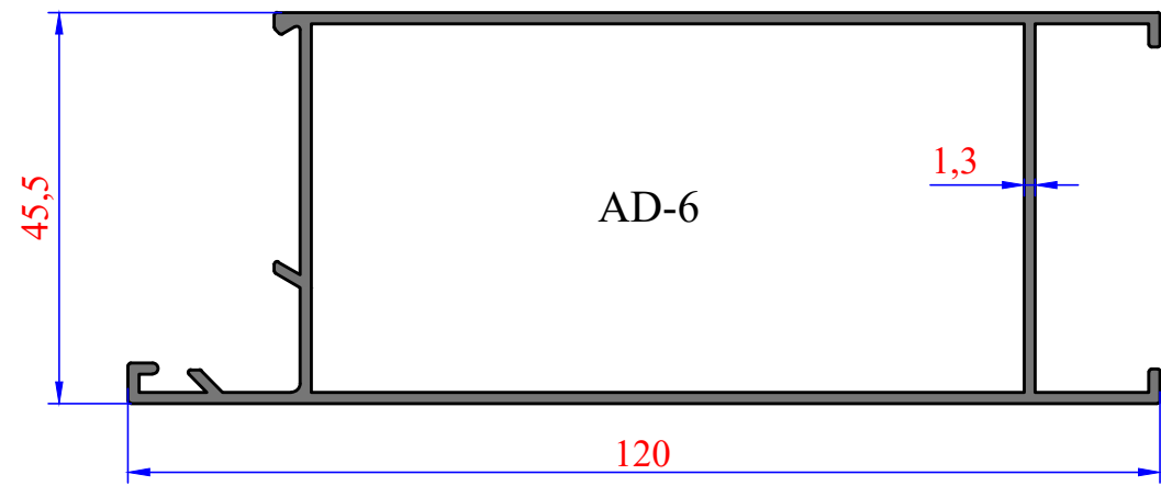
3938 1,157 kg/m ALDOKS ETEK
