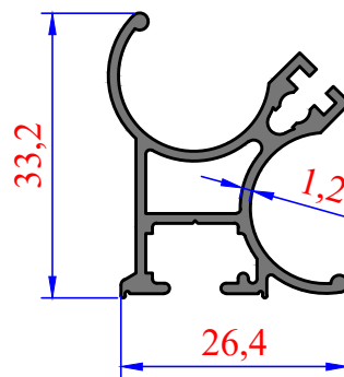
3501 0,431 kg/m Bella Seri
