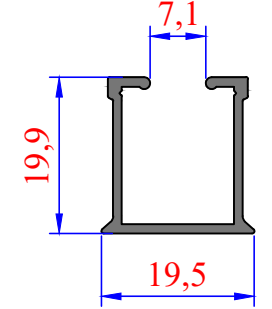
3836 0,208 kg/m
