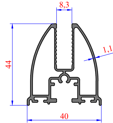
3203 0,763 kg/m Firtına Baza
