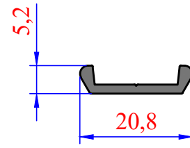
3900 0,124 kg/m
