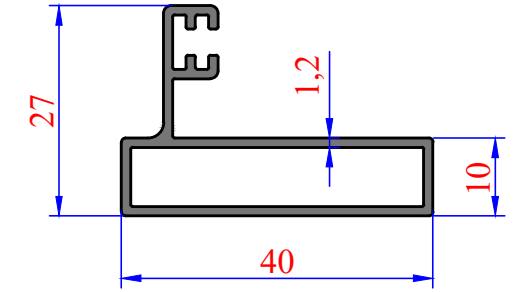
3205 0,426 kg/m 10'luk Dikme
