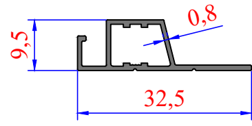
3336 0,159 kg/m
