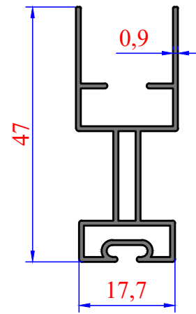
3968 0,392 kg/m 19'luk Plice Kanat
