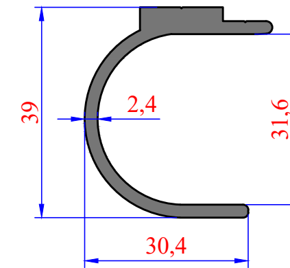
3051 0,651 kg/m 3cm'lik Rustik Ayağı
