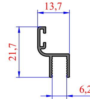
3631 0,142 kg/m 6mm Küçük H
