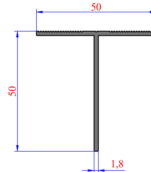
3215 0,461 kg/m
