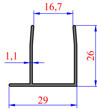
3999 0,234 kg/m Lüks Seri
