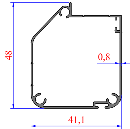
3338 R 0,418 kg/m
