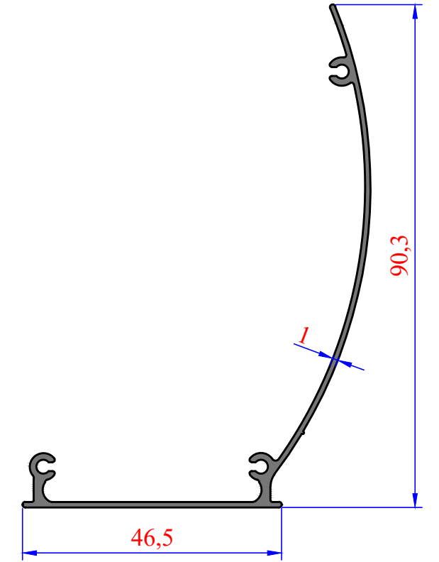
3079 0,499 kg/m
