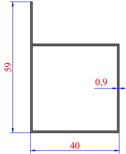
3401 0,404 kg/m
