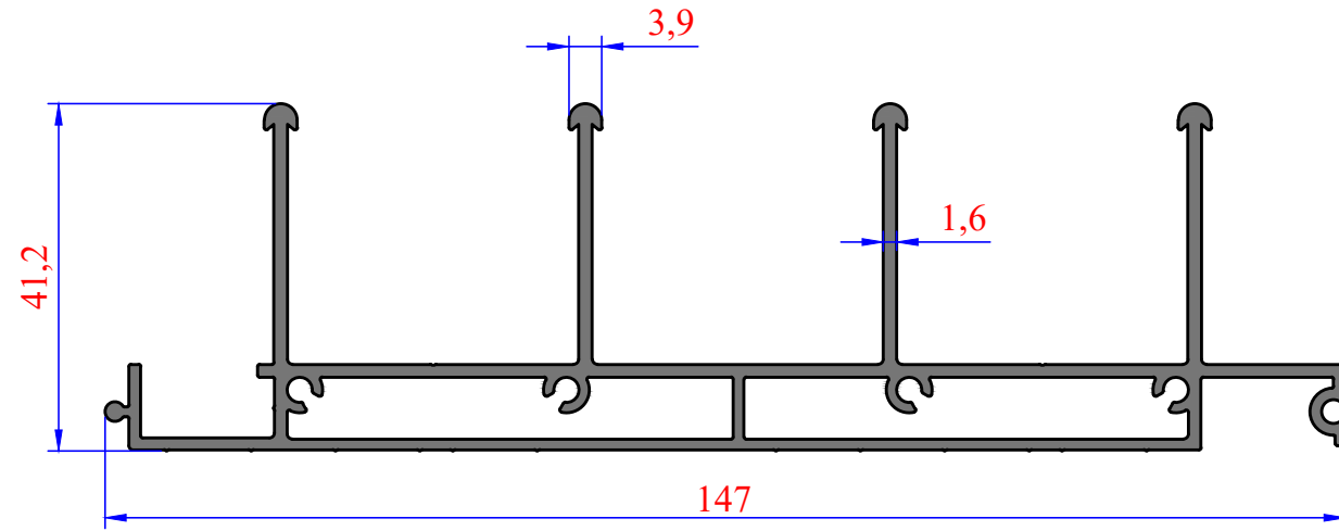
3908 1,816 kg/m
