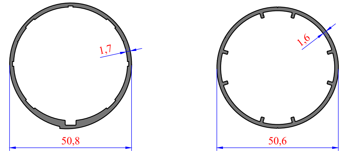
3109 0,772 kg/m
