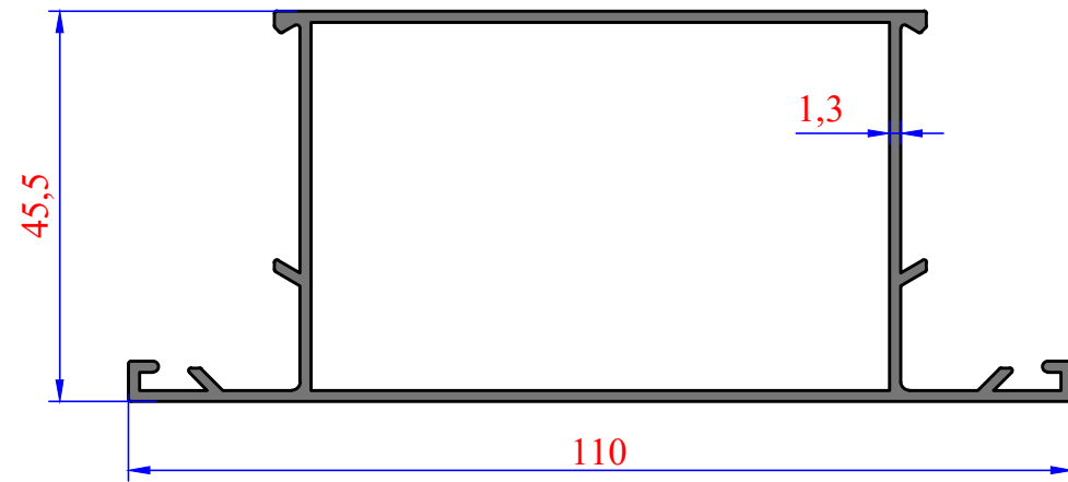
3940 1,029 kg/m GENİŞ ORTA KAYIT
