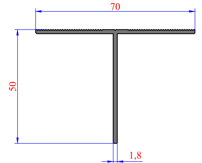
3216 0,547 kg/m
