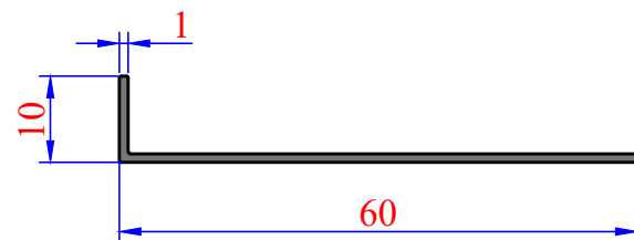
3471 0,187 kg/m
