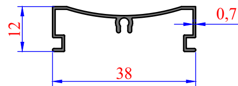
3029 0,157 kg/m Kulaksız Dar Stor Kasa
