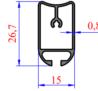
3005 0,237 kg/m Kanallı Lama
