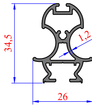
3500 0,484 kg/m Bella Seri
