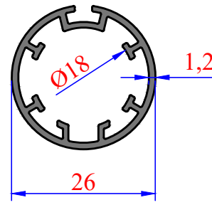
3858 0,348 kg/m
