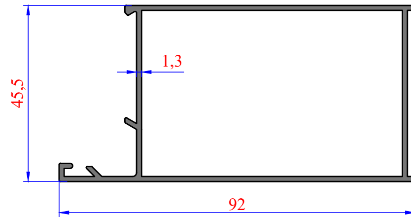
3941 911 kg/m GENİŞ KASA
