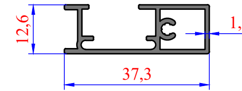
3495 0,329 kg/m Bella Seri
