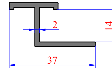
3213 0,347 kg/m
