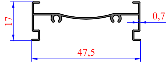
3016 0,204 kg/m Geniş Stor Kasa
