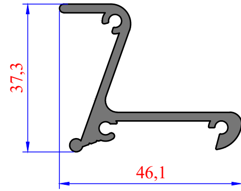
3682 0,698 kg/m Sürme Kilit 1
