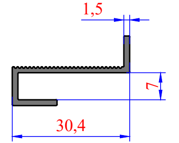
3211 0,218 kg/m
