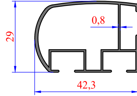
3066 0,438 kg/m
