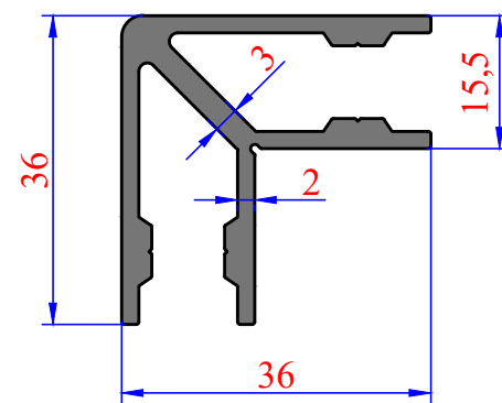
3650 0,858 kg/m AD 4 KÖŞE
