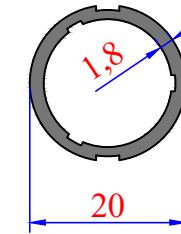
3236 0,260 kg/m
