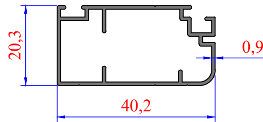
3437 0,351 kg/m
