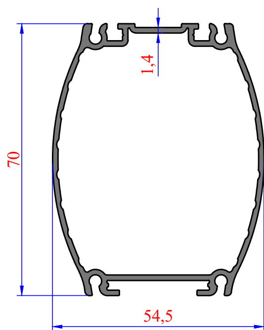
3102 0,978 kg/m
