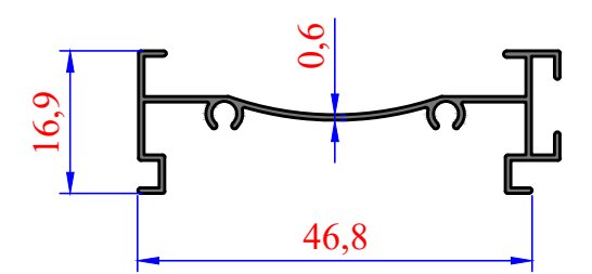
3030 0,213 kg/m Zebra Geniş Kasa 10mm
