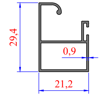
3266 0,266 kg/m
