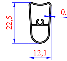
3028 0,144 kg/m Kanalsız Minyatür Lama
