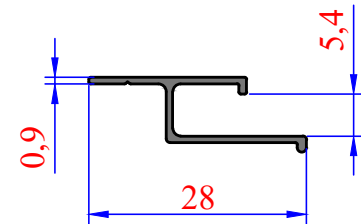
3456 0,111 kg/m Gergi Tavan
