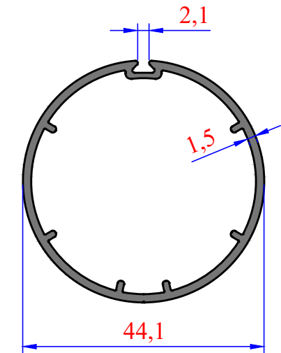
3053 0,594 kg/m
