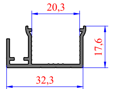
3909 0,304 kg/m
