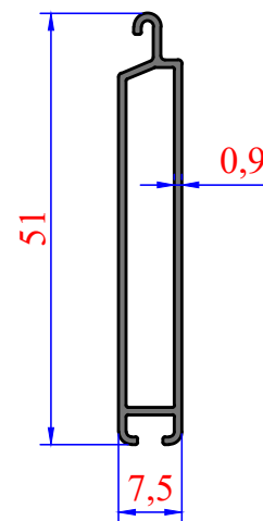
3966 0,272 kg/m
