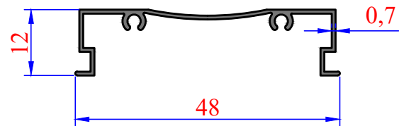
3027 0,182 kg/m Kulaksız Geniş Stor Kasa
