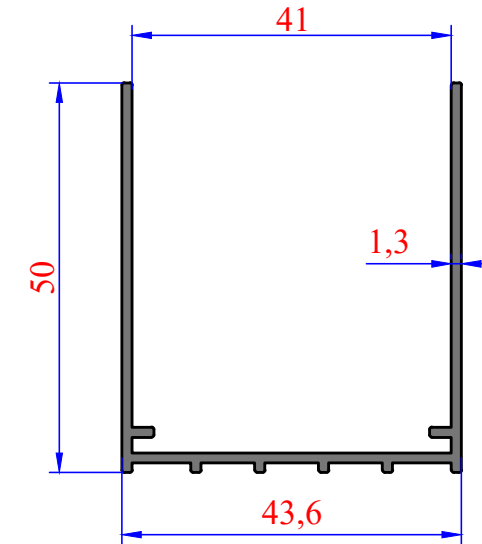
3388 0,532 kg/m
