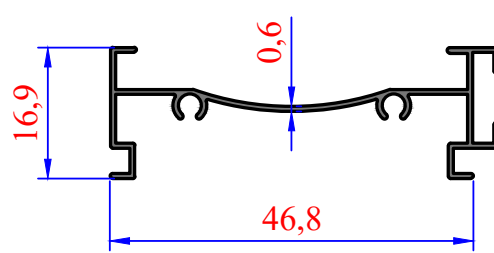
3030 0,213 kg/m Zebra Geniş Kasa 10mm
