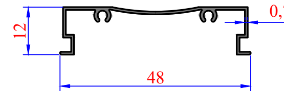
3027 0,182 kg/m Kulaksız Geniş Stor Kasa
