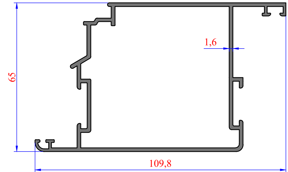
3441 1,534 kg/m SİSTEM GENİŞ KAPI
