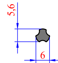
3018 0,060 kg/m Dikey Tül Mili
