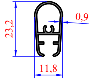
3007 0,178 kg/m Minyatür Lama
