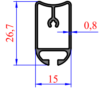
3005 0,237 kg/m Kanallı Lama
