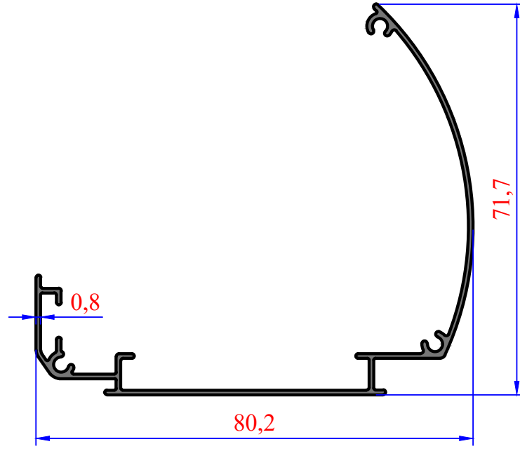
3008 0,498 kg/m Kapalı Kasa
