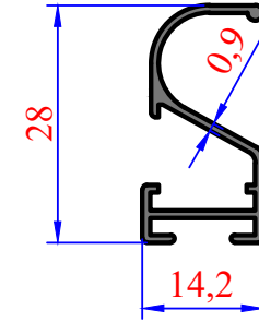
3014 0,187 kg/m Plicel 14'lük Alt
