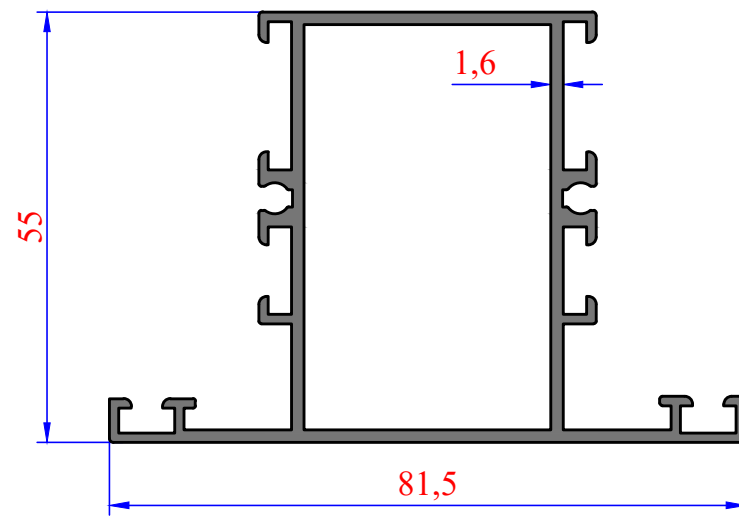
3446 1,221 kg/m SİSTEM 2 ORTA KAYIT
