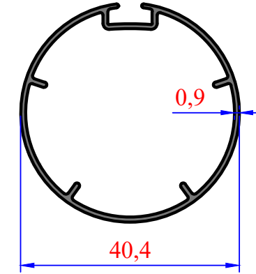
3004 0,360 kg/m 38'lik Jumbo Tırnaklı Boru
