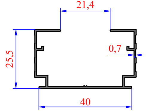
3022 0,298 kg/m Dikey Tül Kasa
