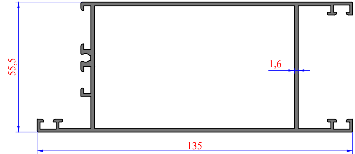
3440 1,725 kg/m SİSTEM 135'lik ETEK
