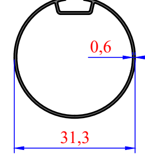
3002 0,180 kg/m 32'lik Stor Boru
