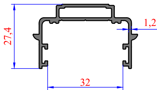
3640 0,463 kg/m Isıcamlı Surme Kulp Bağlantı
