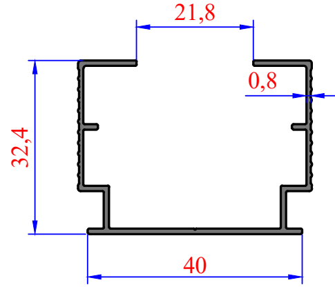
3032 0,357 kg/m Dikey Tül Kasa
