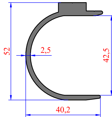
3052 0,880 kg/m 4cm'lik Rustik Ayağı
