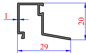
3454 0,193 kg/m AD ISI CAM ÇITA
