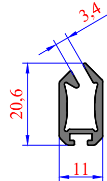
3044 0,233 kg/m Özel Lama
