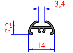
3060 0,095 kg/m Açık Kasa
