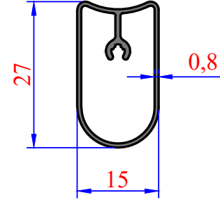
3017 0,187 kg/m Düz Kanalsız Lama
