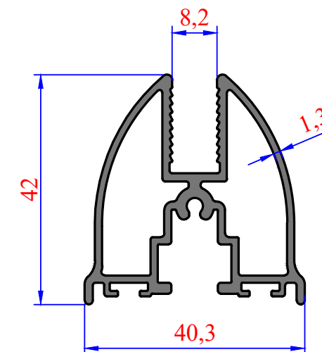
3253 0,875 kg/m Gold Baza
