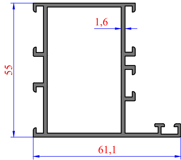
3443 1,068 kg/m SİSTEM 5 KASA
