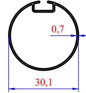
3011 0,196 kg/m 30'luk Stor Boru
