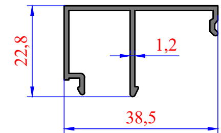
3445 0,304 kg/m SİSTEM TEK CAM ÇITA
