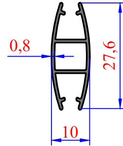
3034 0,168 kg/m Stor Etek Çıtası
