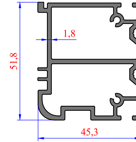
3637 1,371 kg/m SİSTEM 55 ADAPTÖR
