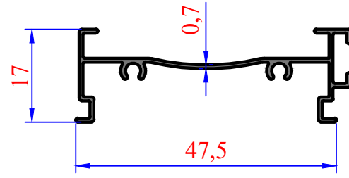
3003 0,233 kg/m Zebra Geniş Kasa
