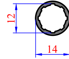
3006 0,140 kg/m 8'li Boş Mil
