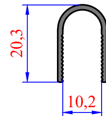
3602 0,154 kg/m 10mm U Fitol
