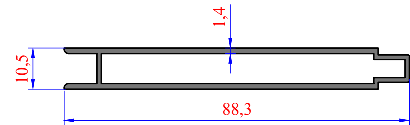
3572 0,706 kg/m TAHTA LAMBRI
