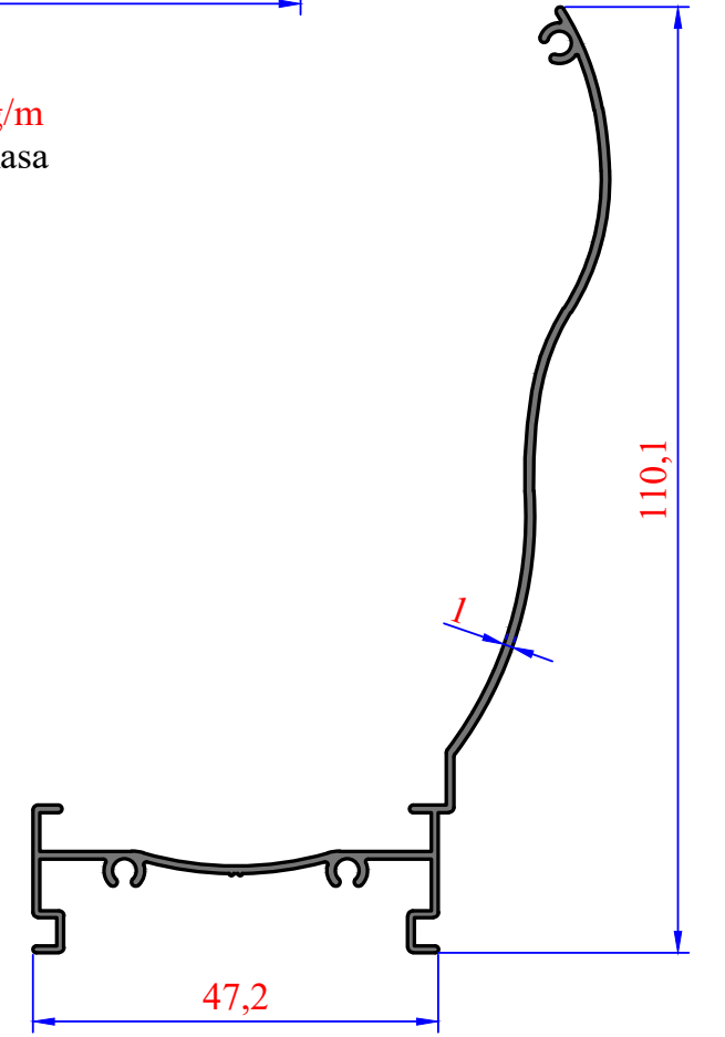
3020 0,541 kg/m Çiftli Kapalı Kasa
