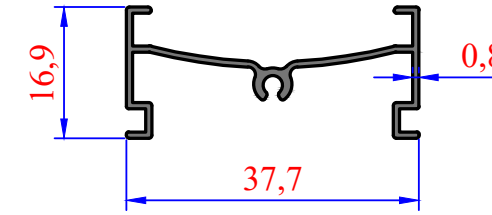
3001 0,207 kg/m Dar Stor Kasa
