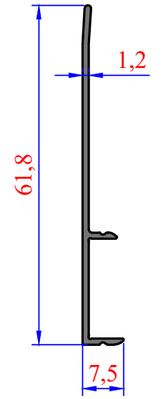
3599 0,222 kg/m U Ayar Kapak
