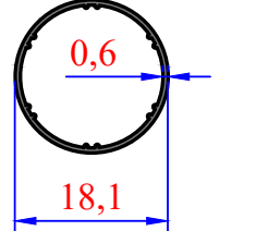
3058 0,095 kg/m 18'lik Boru
