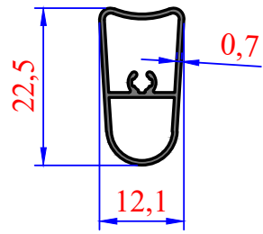
3028 0,144 kg/m Kanalsız Minyatür Lama
