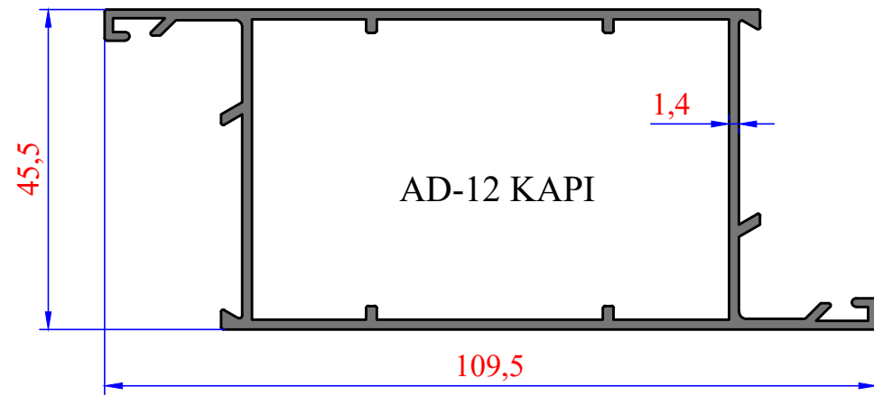
AD-12 KAPI 3400 1,153 kg/m AD GENİŞ KAPI
