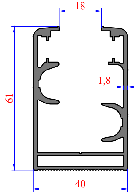
3202 1,255 kg/m Firtina Kasa
