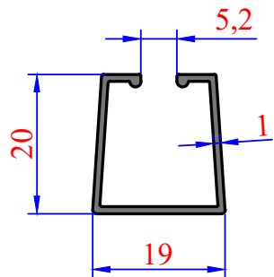
3035 0,184 kg/m Rustik Ray
