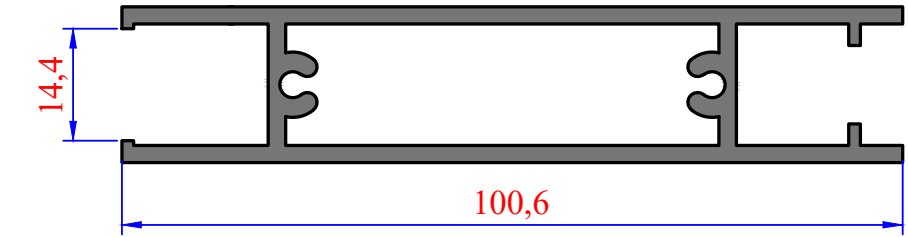
3574 1,541kg/m Fotosel Etek Üst
