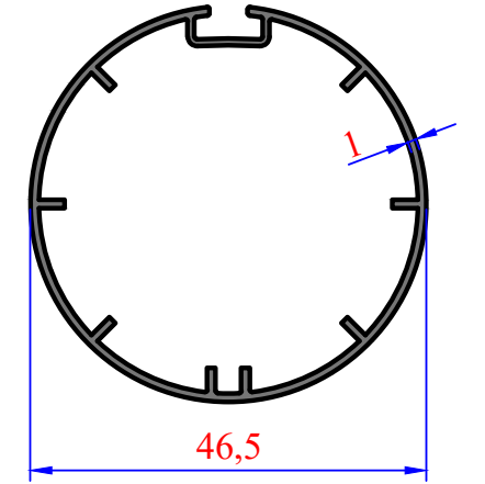
3013 0,470 kg/m 47'lik Motor Boru
