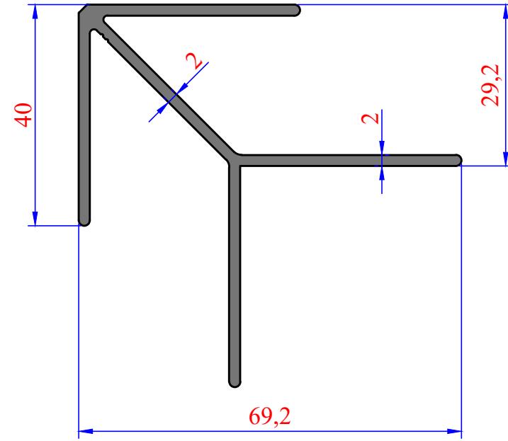
3648 1,056 kg/m SİSTEM KÖŞE
