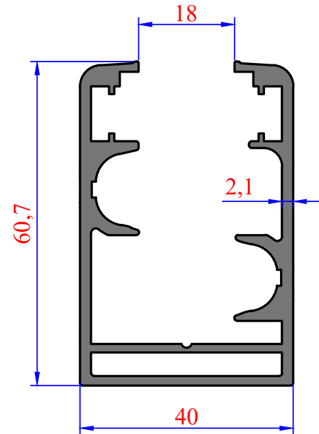
3256 1,464 kg/m Firtina Kasa
