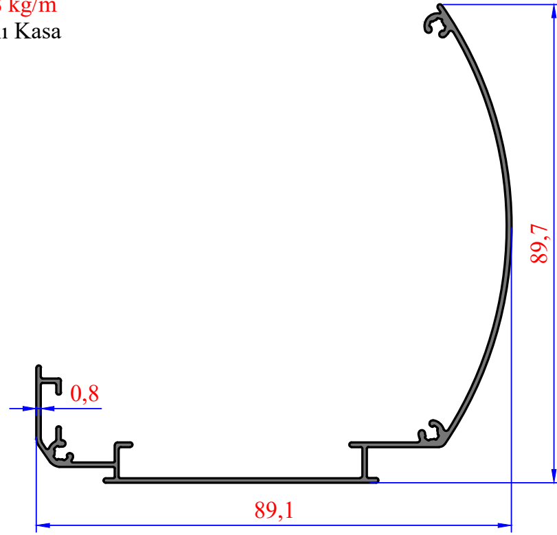
3019 0,567 kg/m 12'lik Jumbo Kapalı Kasa
