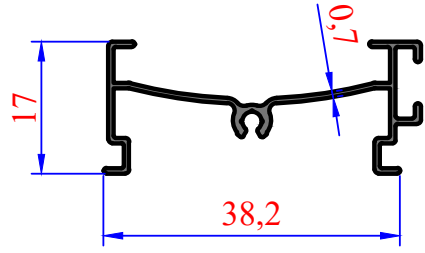
3010 0,204 kg/m Zebra Dar Kasa
