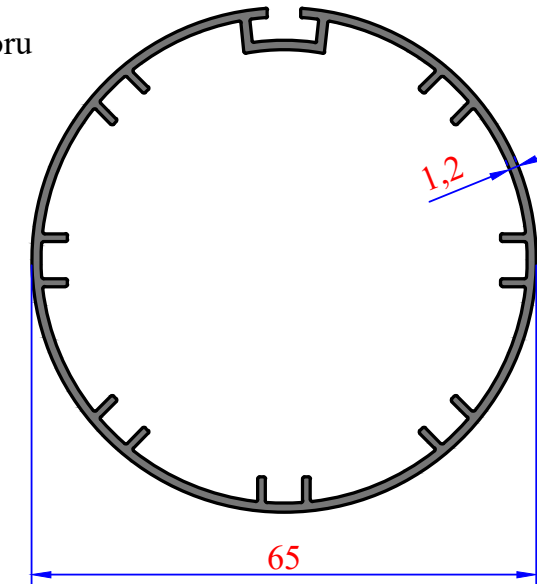
3033 0,815 kg/m 65'lik Motor Borusu
