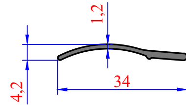
3068 0,130 kg/m Yan Kayıt
