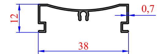
3029 0,157 kg/m Kulaksız Dar Stor Kasa
