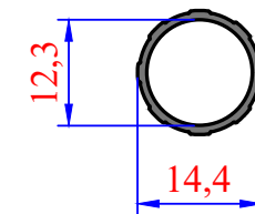
3050 0,106 kg/m Tırtıklı Boş Mil
