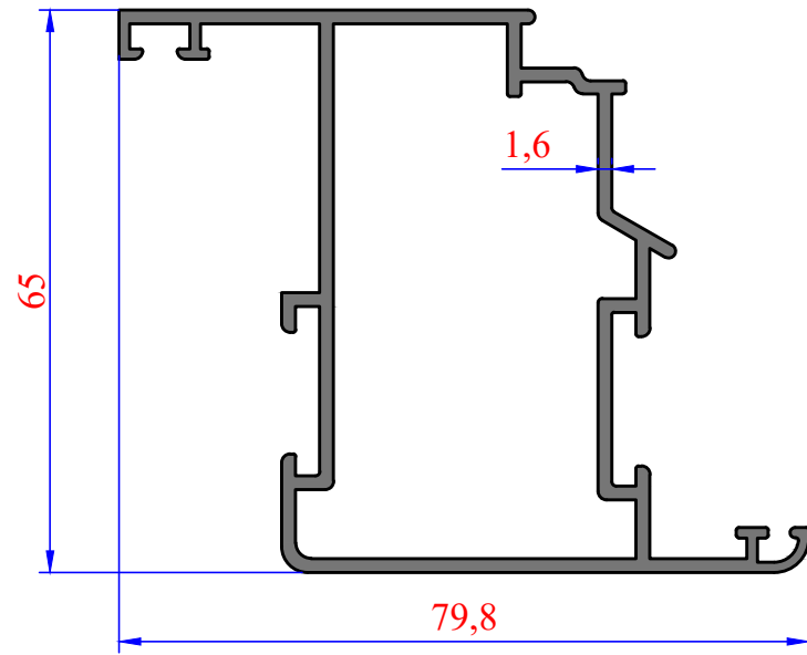
3442 1,267 kg/m SİSTEM PENCERE KANAT
