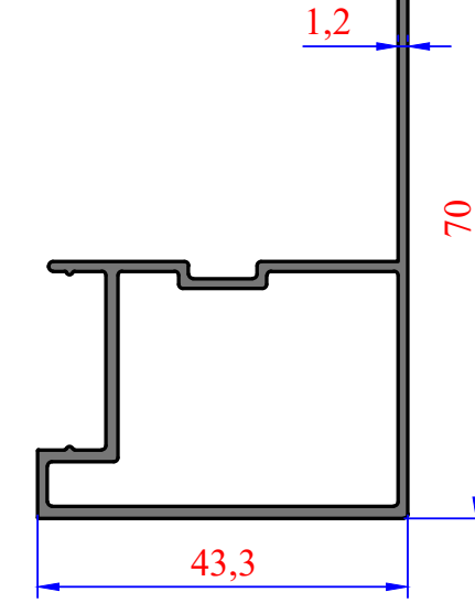
3598 0,650 kg/m U Ayar
