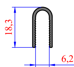
3632 0,131 kg/m 6mm U Fitol
