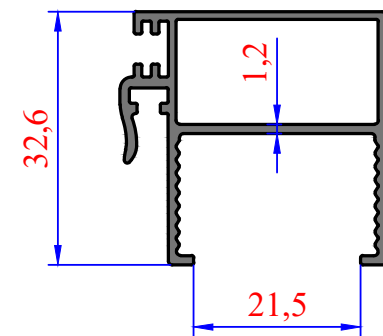
3641 0,459 kg/m Isıcamlı Surme Çekme Çita Profili
