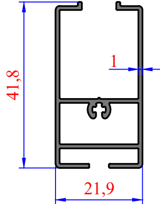
3043 0,444 kg/m Özel Lama
