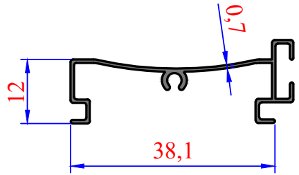
3038 0,177 kg/m Alınsız Zebra Dar Kasa
