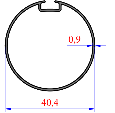
3037 0,325 kg/m 38'lik Jumbo Tırnaksız
