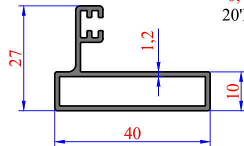
3205 0,426 kg/m 10'lik Dikme
