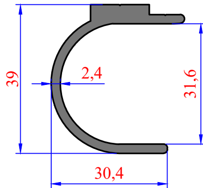
3051 0,651 kg/m 3cm'lik Rustik Ayağı
