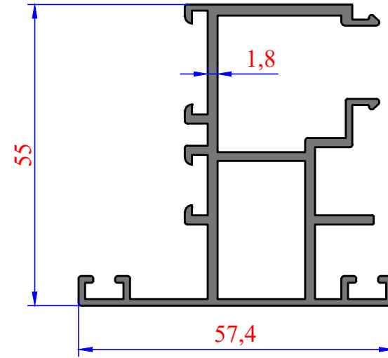
3444 1,107 kg/m SİSTEM ÇİFT KAPI ADAPTÖR
