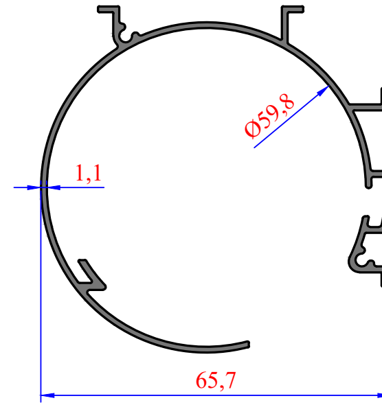
3040 0,705 kg/m Stor Kapalı Kasa
