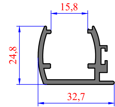
3577 0,502kg/m Fotosel Fitol Arka
