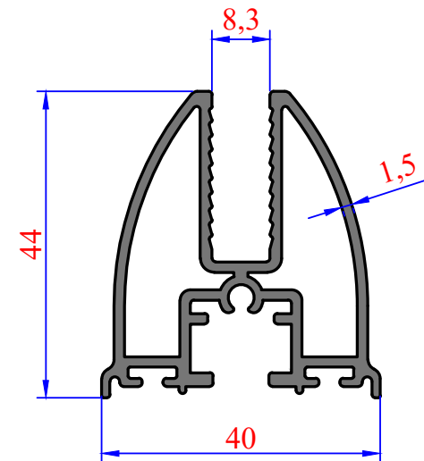
3257 0,990 kg/m Firtina Baza
