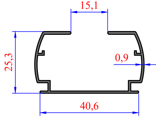
3021 0,325 kg/m Dikey Tül Kasa
