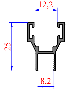
3240 0,220 kg/m Büyük H
