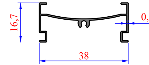
3048 0,172 kg/m İnce Dar Stor Kasa
