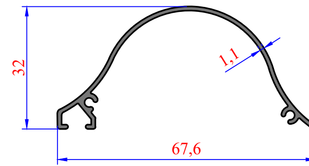
3061 0,361 kg/m Mini Kapalı Kasa
