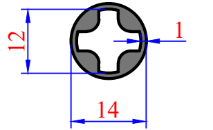
3012 0,209 kg/m Artı mil
