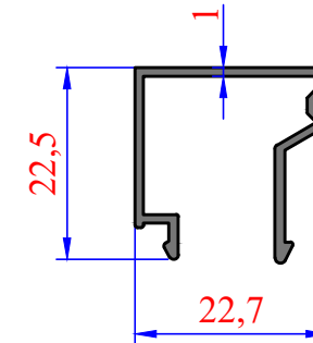
3570 0,217 kg/m SİSTEM ISI ÇITA
