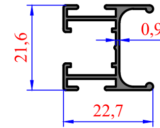
3015 0,244 kg/m Plicel 14'lük Orta
