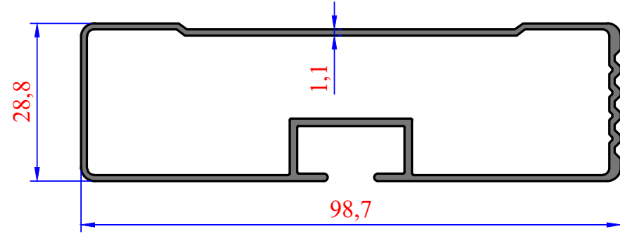
3518 0,904 kg/m 100'lük Bisikletlik
