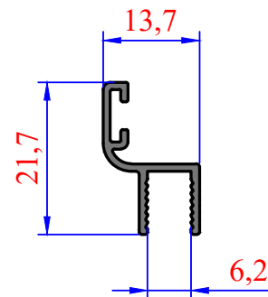
3631 0,142 kg/m 6mm Küçük H
