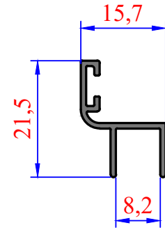
3241 0,141 kg/m Küçük H
