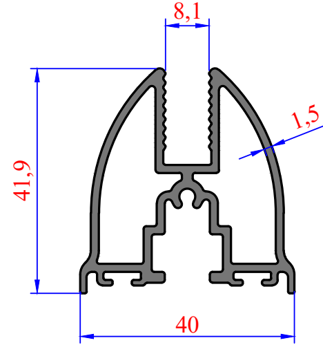
3264 0,929 kg/m Gold Baza
