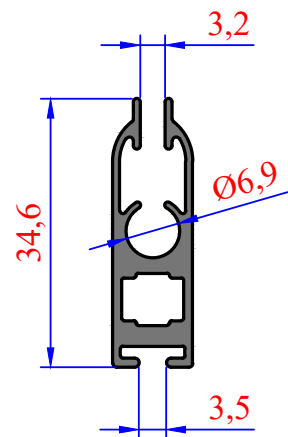
3554 0,384 kg/m Lazer Perde Laması
