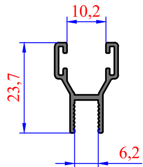
3630 0,202 kg/m 6mm Büyük H
