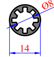
3009 0,193 kg/m Yıldız Mil
